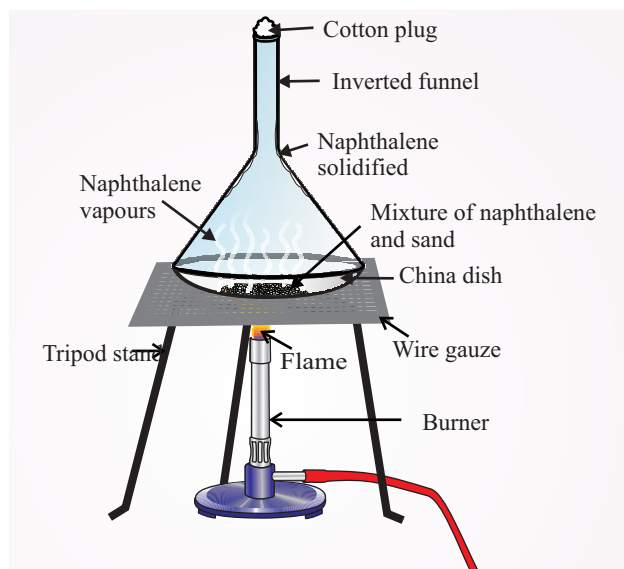
Fig. 12.6 : Sublimation
