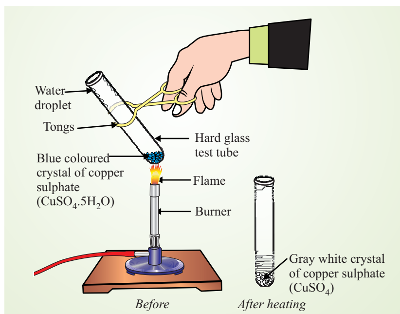
Fig. 14.2 Heating of \text{CuSO}_4 \cdot 5\text{H}_2\text{O}
